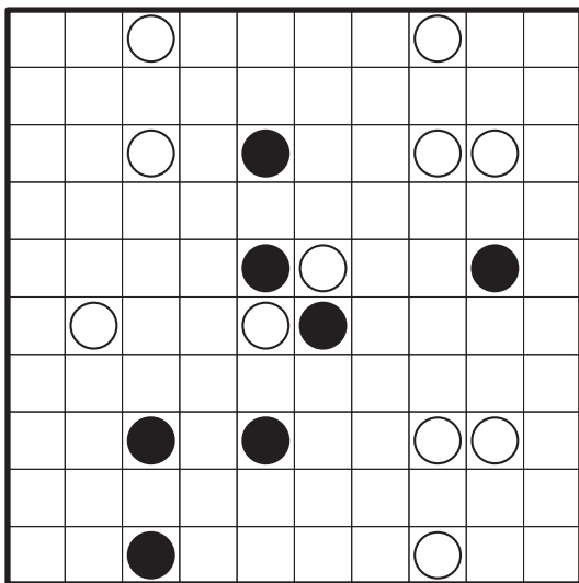
Masyu
